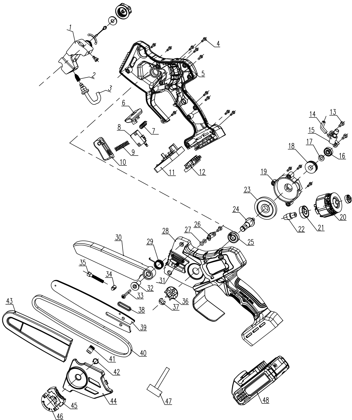
YMCA1801爆炸图
